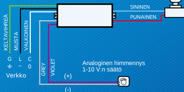
Johdotuskaavio:
